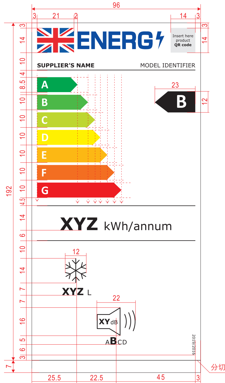
尺寸定位示意图
